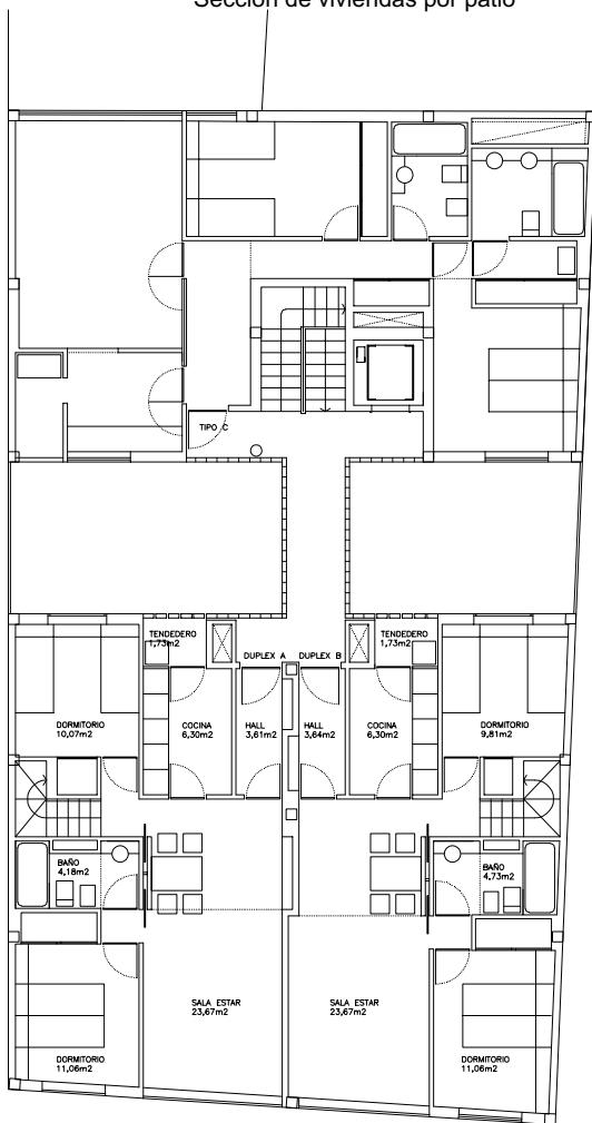
Seccion de viviendas por patio
