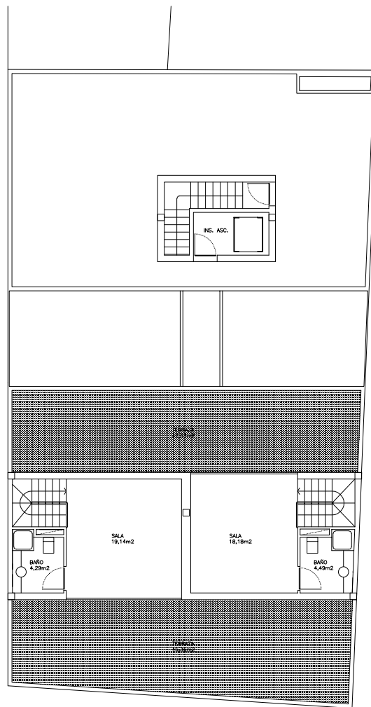
VIVIENDAS DUPLEX (ÁTICO) PLANTA CUBIERTAS cota +17.28 e1/50
